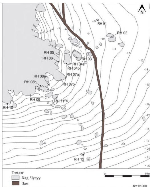
Рашаан хадны дэвсгэр зураглал
