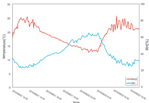
Зураг 1. Рашаан хадны хүрээлэн буй орчны чийгшил дулааны хэмжилт
