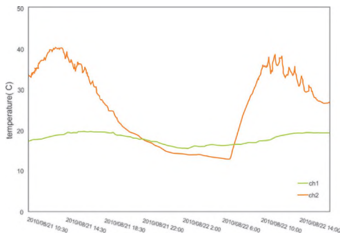
зураг 2. Рашаан хадны чулуулгийн гадаргууд хийсэн дулааны хэлбэлзэл болон усны агууламжийн хэмжилт
